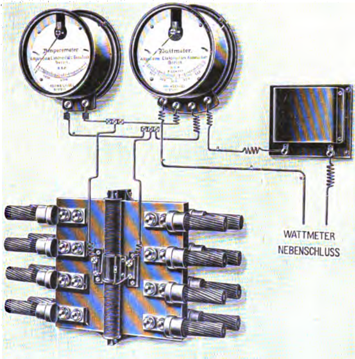
Abb. 465. Stromwandler der Allgem. Elektr.-Ges. mit Schienenstück.
